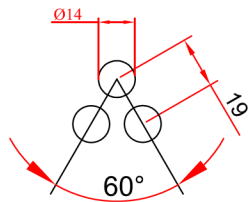
Detalj "A"
